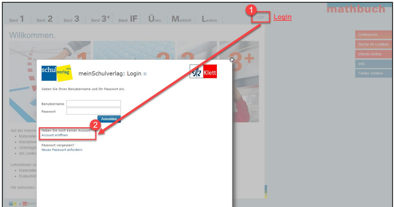
Abbildung 1: Account eröffnen
